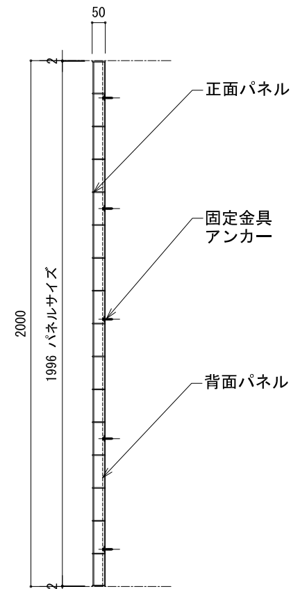
断面図
